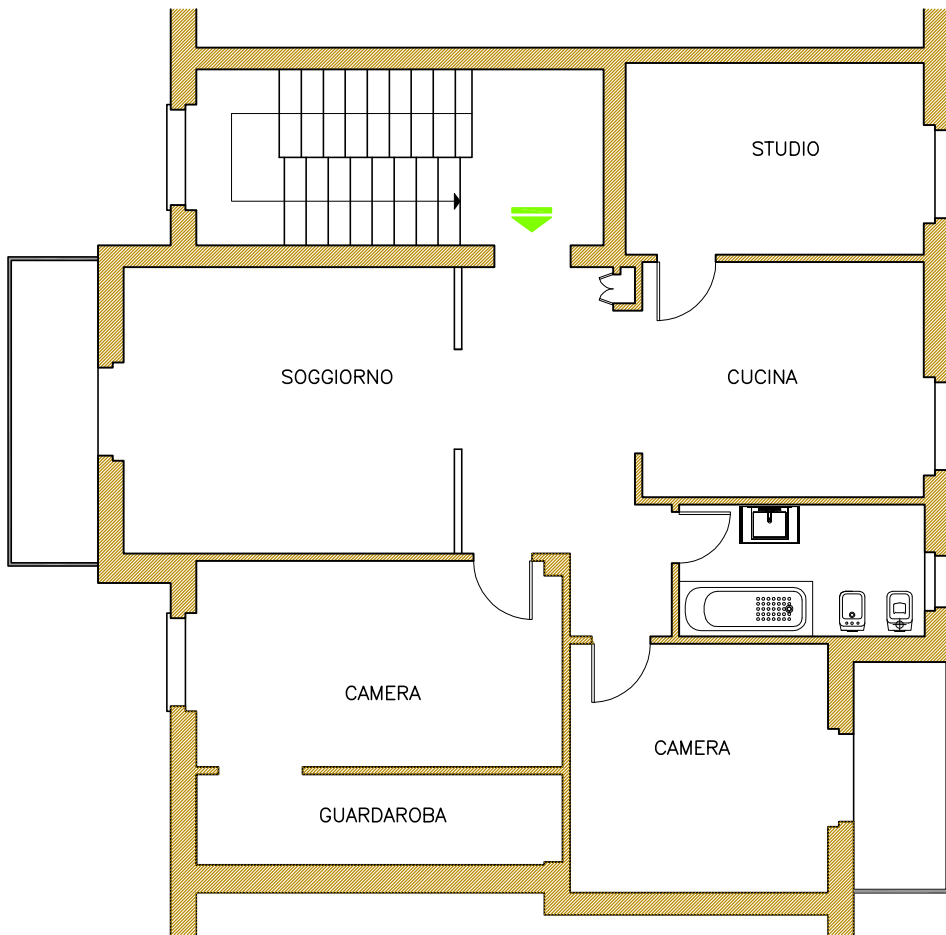
PIANTA STATO REALIZZATO Scala 1:100
