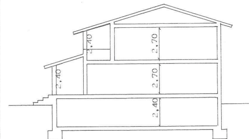
SEZIONE A-B
