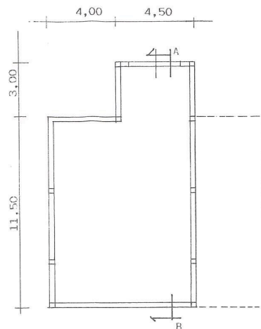
PIANTA PIANO SEMINTERRATO
