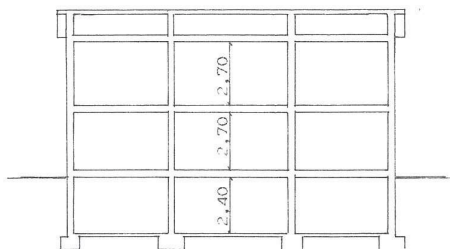
SEZIONE A-B
